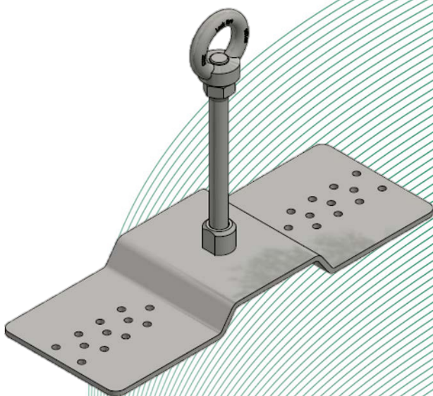
Bild 1: Anschlageinrichtung, Typ: ABS-Lock® X-SW-6
