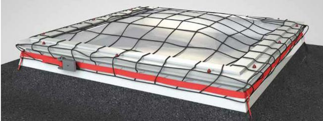
Photo 1: Protection antichute avec dispositif d'ancrage, type ABS DomeWeb
