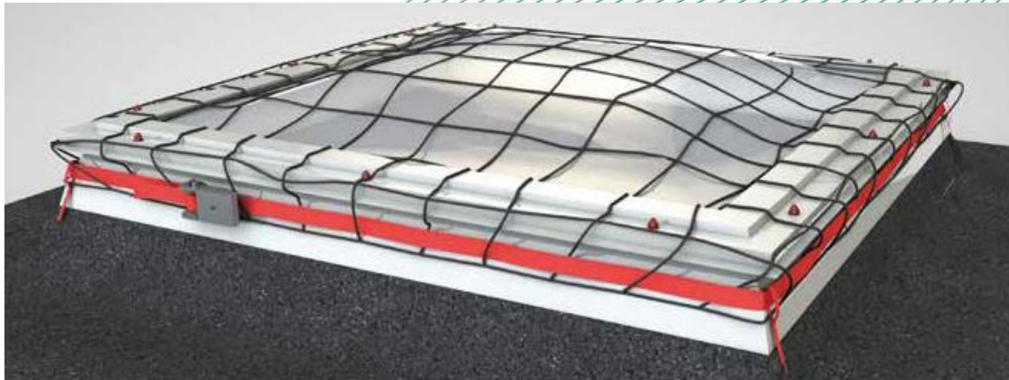
Bild 1: Anschlageinrichtung mit Durchsturzsicherung, Typ: ABS DomeWeb
